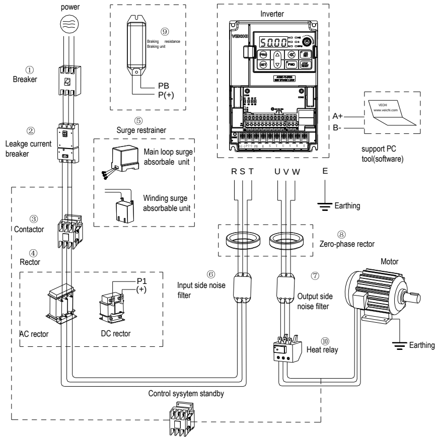
Görsel 9-1: Çevre birimi bağlantıları blok şeması
