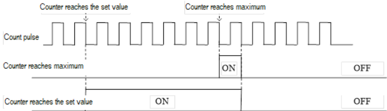
Sayaç maksimum değeri ve sayaç ayar değeri ile ilgili çalışma şeması
