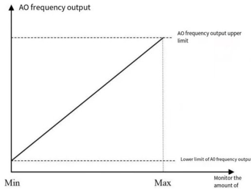
AO bağlantı noktası pals frekansı çıkış şeması
