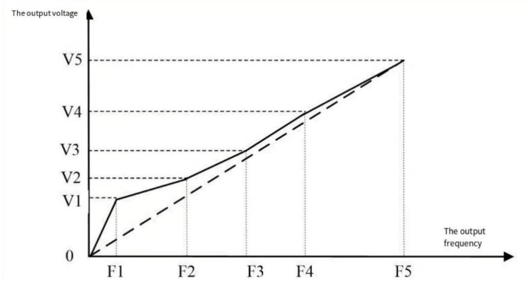
Özel eğri diyagramı
