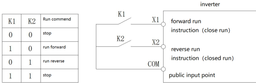
İki kablolu sistem kontrolünün şematik diyagramı 1
