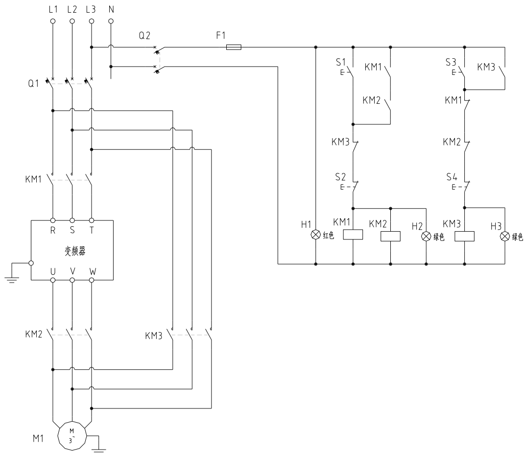
Şekil 3-7: Yedek kontrol sistemi bağlantısı örneği
