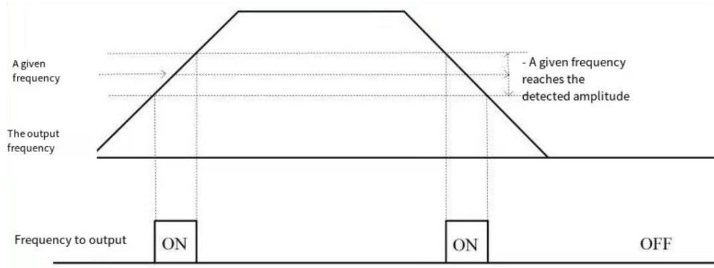
Frekans algılama diyagramı
