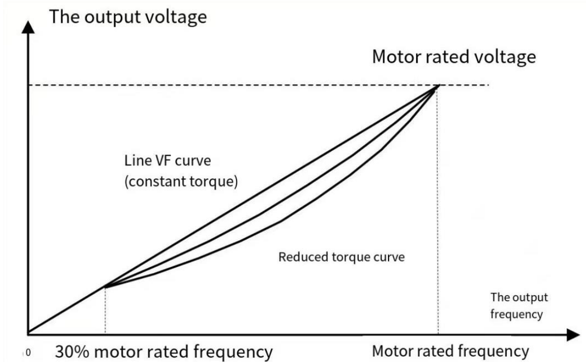
VF çizgisi ve tork azaltma eğrisi
